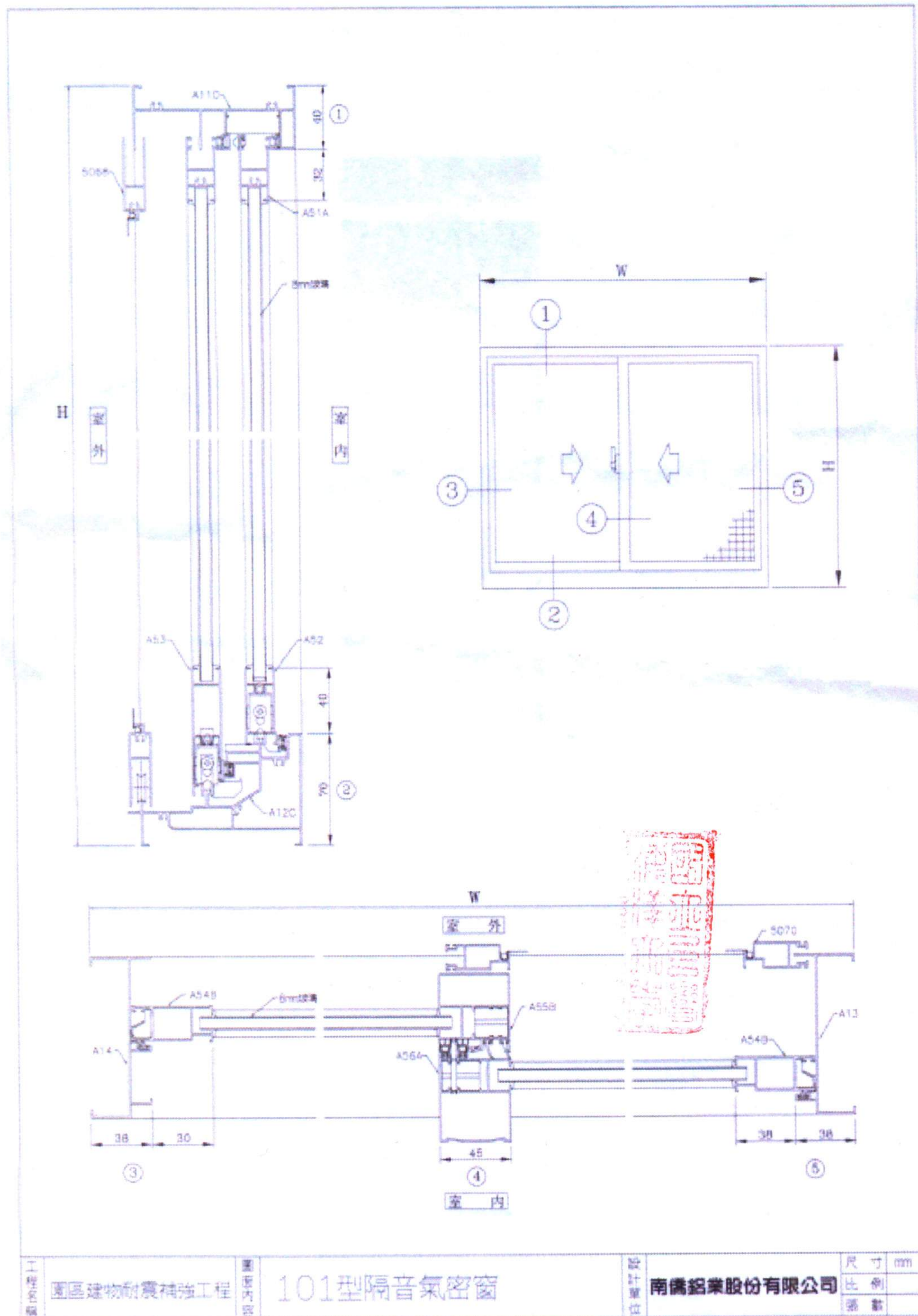
圖 3 試樣結構圖
